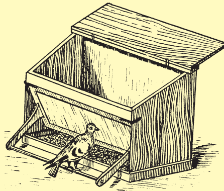
Selbsttätiger Futterkasten
